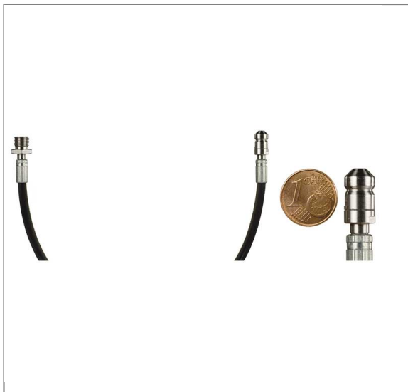
Mini-Rohrreinigungsleitung mit Düse
